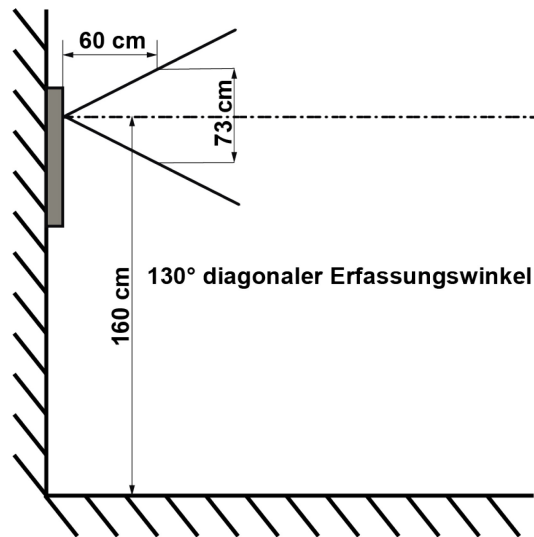
Abb. 6: Montagehöhe Video-Außenstation
