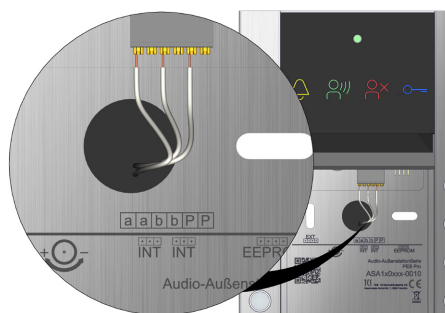
Abb. 15: Anschluss ASA
