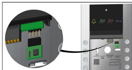
Abb. 25: Backup-EEPROM entfernen
