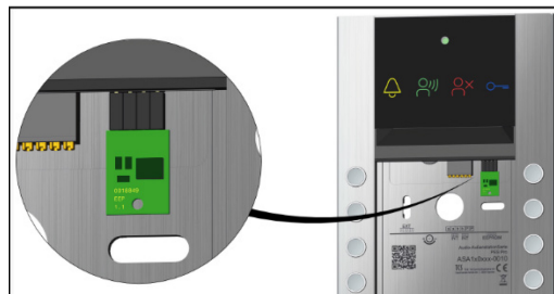
Abb. 24: Alten EEPROM stecken
