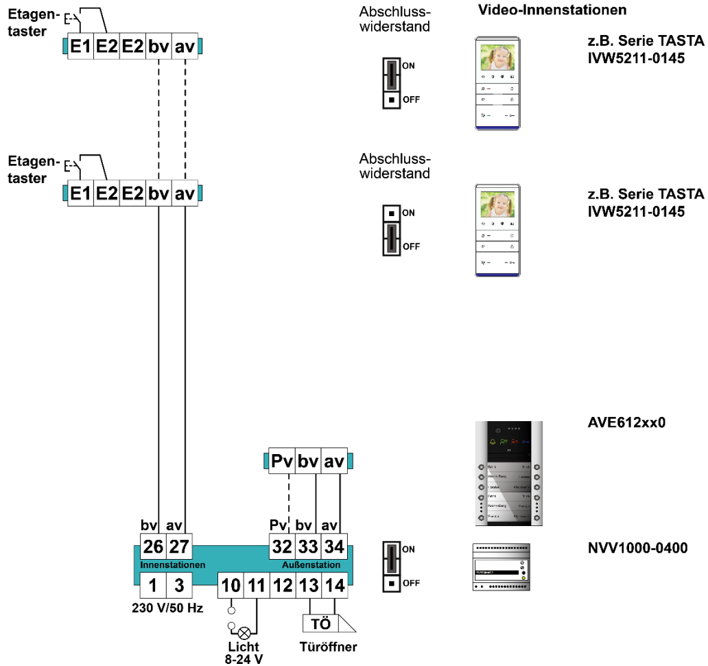
Abb. 19: Schaltungsbeispiel für Video-Außenstation AVA6... Video-2-Draht:BUS
