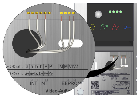
Abb. 16: Anschluss AVA
