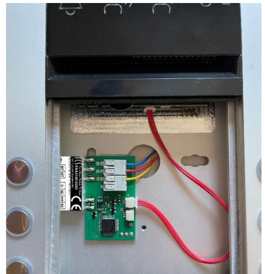
Abb. 20: FAA3100-0300 anschließen
