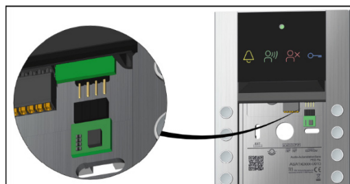
Abb. 23: Backup-EEPROM entfernen
