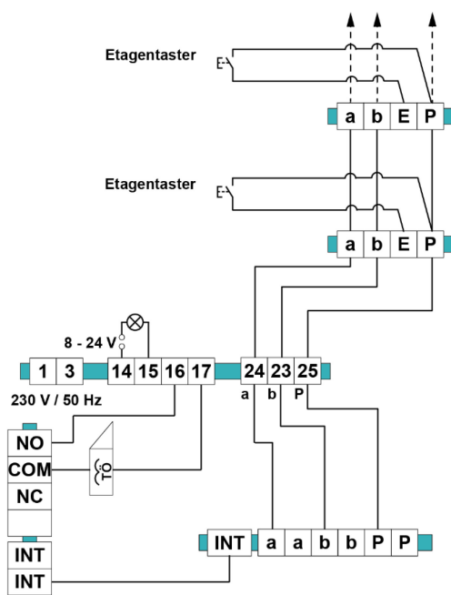
Abb. 21: Schaltplan
