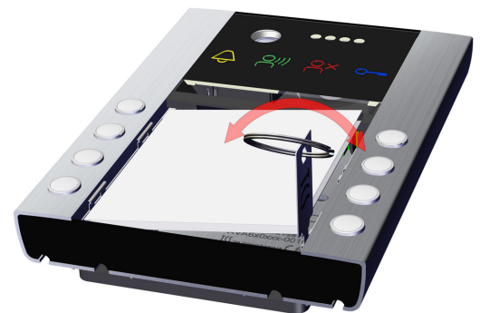
Abb. 9: Entnahmewerkzeug als Hebel benutzen
