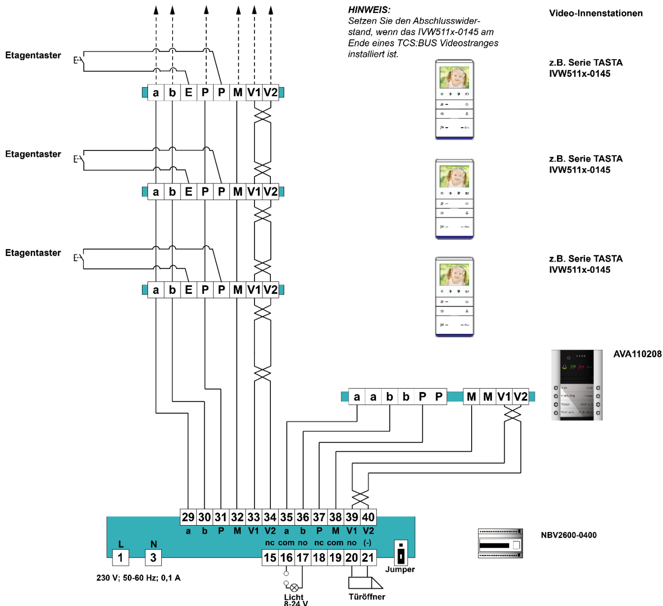
Abb. 18: Schaltungsbeispiel für Video-Außenstation AVA6...
