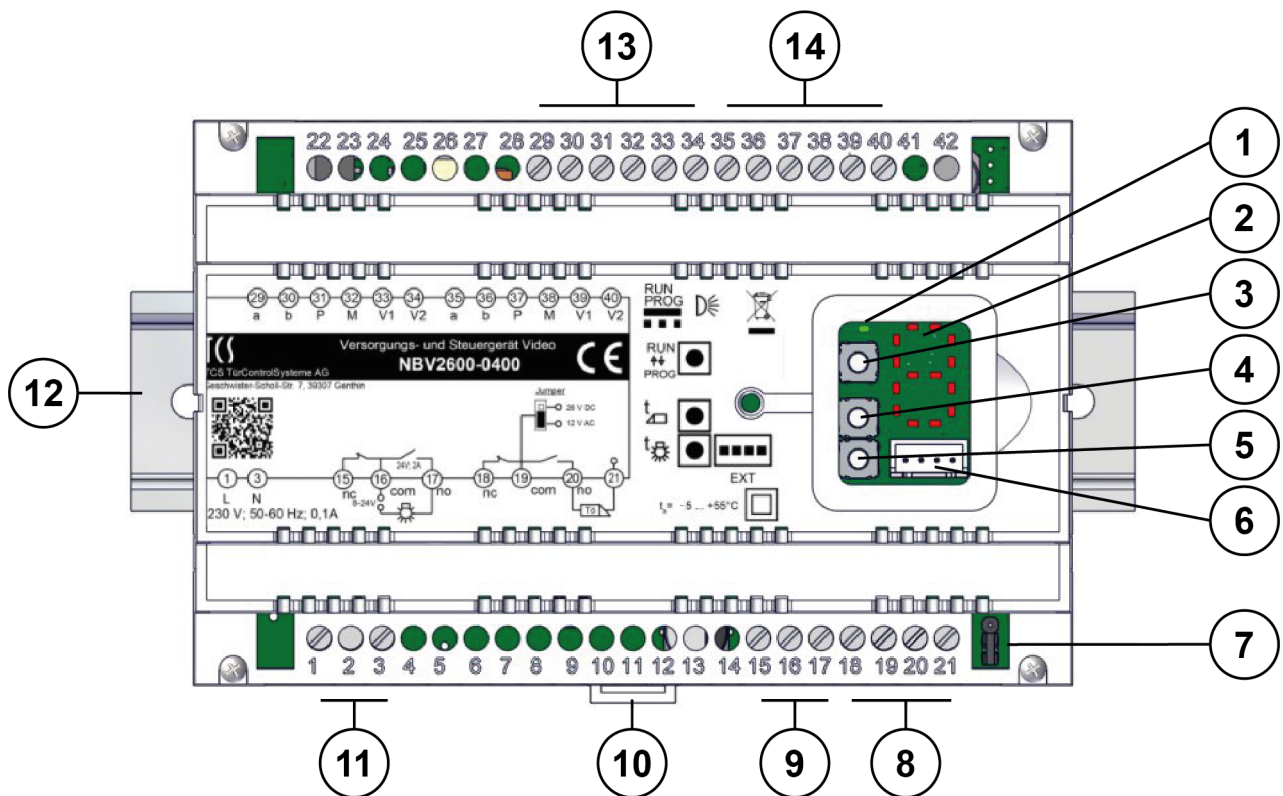
Abb. 1: Geräteübersicht
