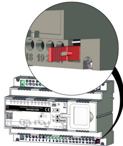
Abb. 8: Türöffnerversorgung AC/DC
