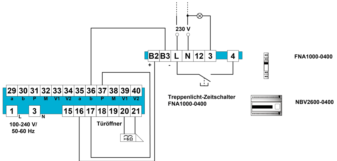
Abb. 6: Schaltungsbeispiel Treppenlicht-Zeitschalter FNA1000-0400
