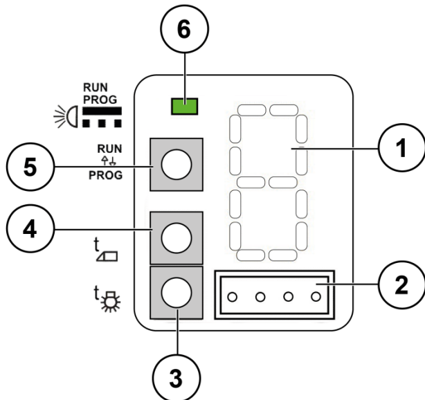
Abb. 7: Serviceöffnung
