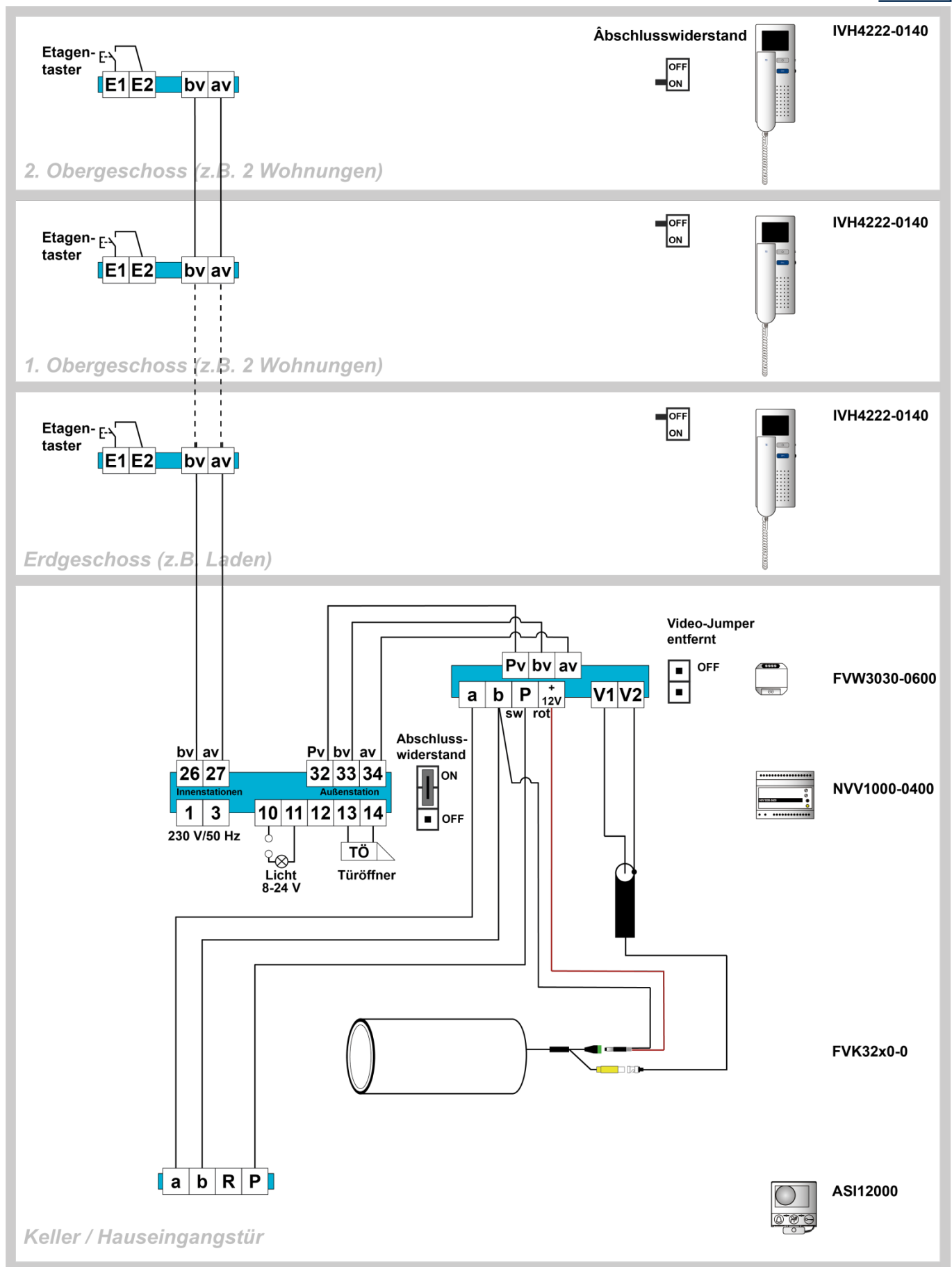
Abb. 7: FVW3030 mit Audio-Außenstation (ASI11000) und FVK3220-0
