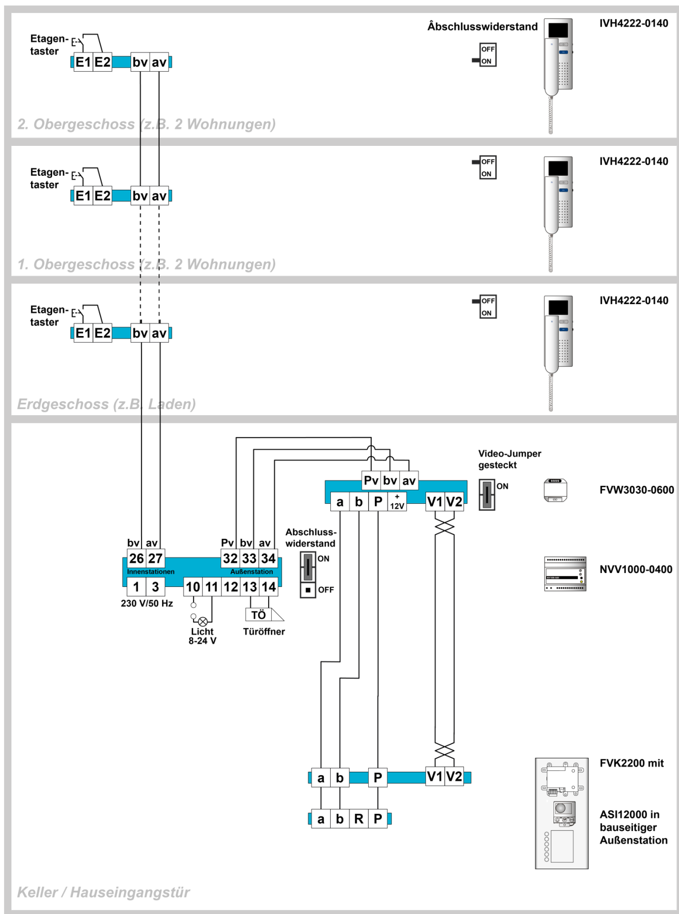
Abb. 6: FVW3030 mit Audio-Außenstation (ASI11000) und FVK2200-0
