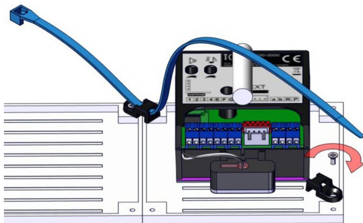
Montage mittels Schraubsockel
