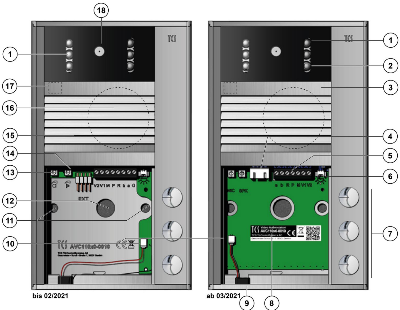
Abb. 1: Geräteübersicht
